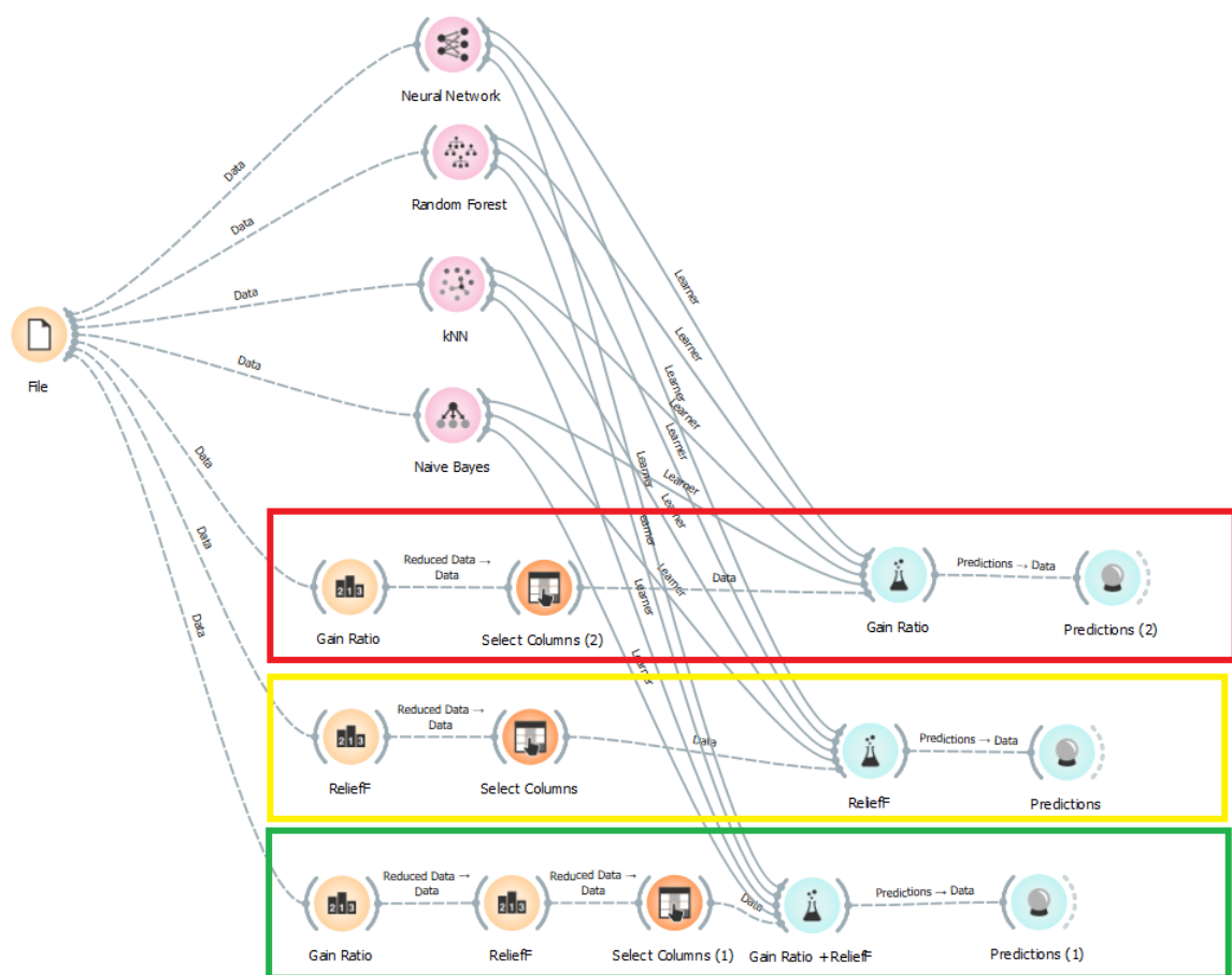
Figura 4.3: Implementação do algoritmo proposto utilizando o framework Orage (Demšar et al., 2013)
