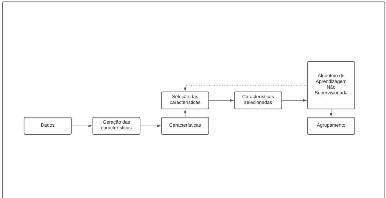
Figura 3.7: Seleção de características em modelos não supervisionados
