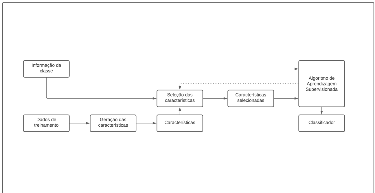
Figura 3.6: Seleção de características em modelos supervisionados
